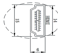
Detail:A Scale 3:1
